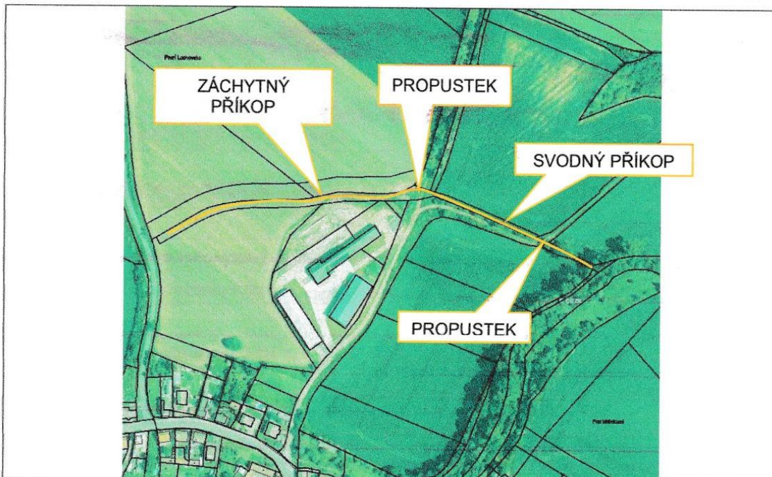
Obr. 29 Návrh záchytného příkopu
